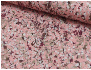
A337G
